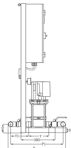
ELINOX-VS, ALTI-VS (2 et 3 pompes) coffret variation de vitesse (CV)
