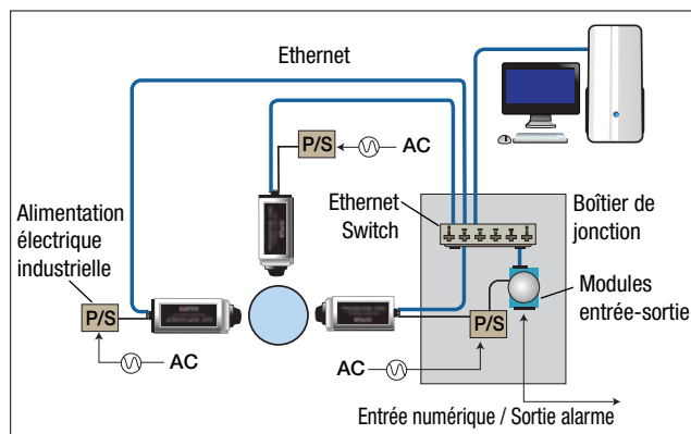
Exemple d'installation avec plusieurs caméras ThermoView Pi20
