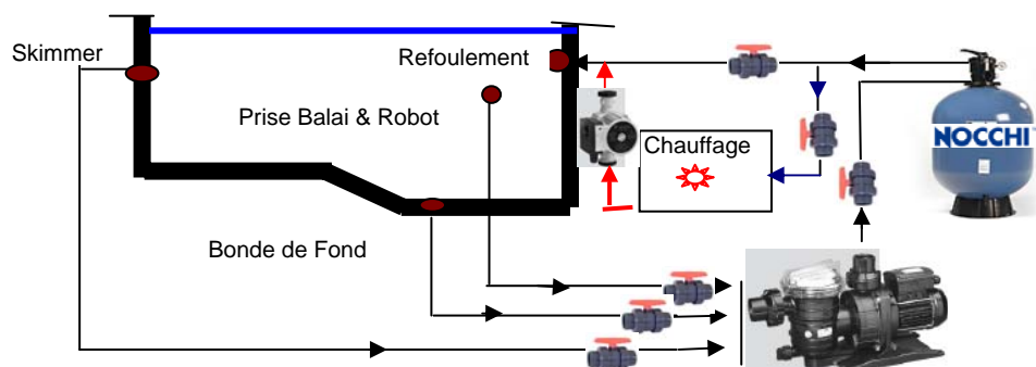
Shéma d'installation
