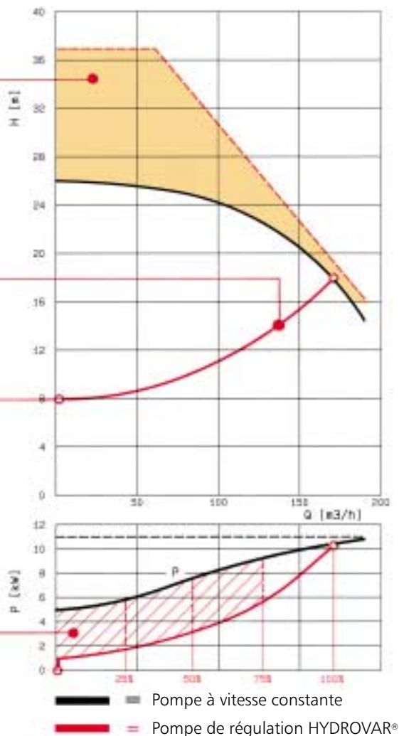
POMPE DE CIRCULATION AYANT UN MOTEUR D'UNE PUISSANCE DE 11 KW SOUS CHARGE PARTIELLE
