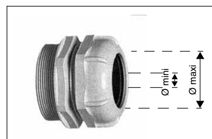
Presse-étoupe polyamide
