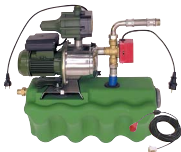
CENTRALE DE PILOTAGE avec flotteur - Code 355002
