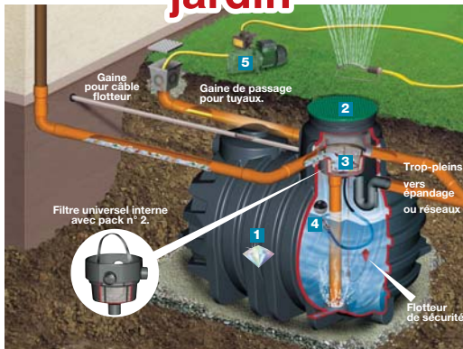
EXEMPLE D'INSTALLATION JARDIN (Cuve avec couvercle et Pack N° 2)
