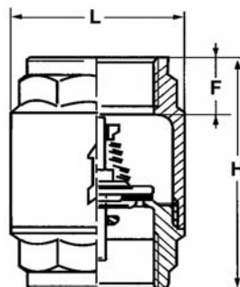
Clapets 303 et 305
