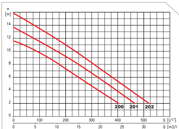
Courbes hydrauliques
