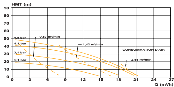
Modèle AOD - 1 1/2" Membranes Elastomères
