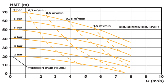
Modèle AOD - 1"
