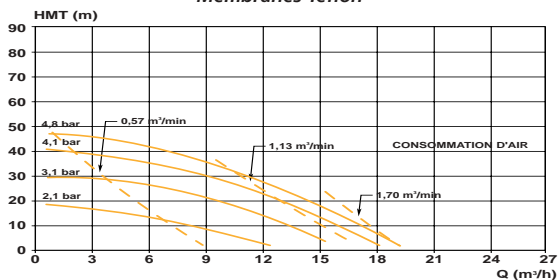
Modèle AOD - 1 1/2" Membranes Teflon
