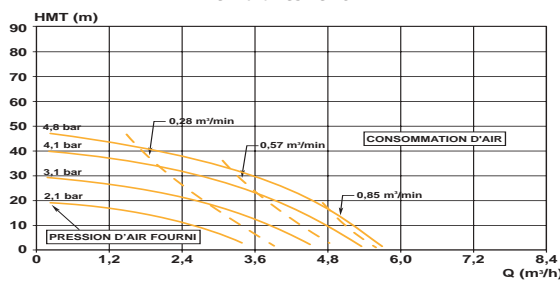
Modèle AOD - 3/4" Membranes Teflon
