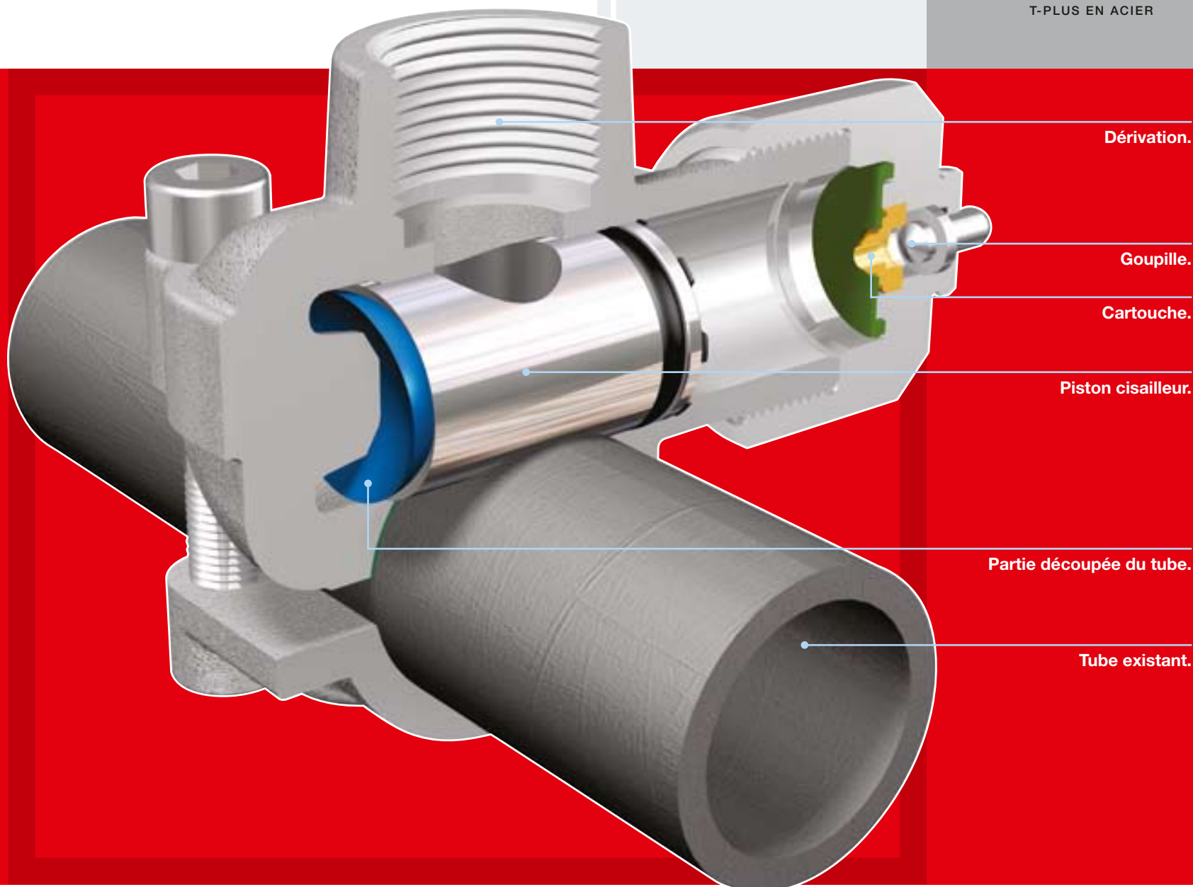
T-PLUS EN ACIER
