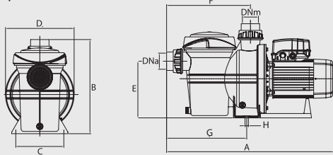
▼ dimensions
