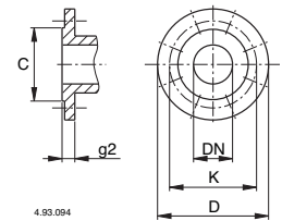
Brides EN 1092-2
