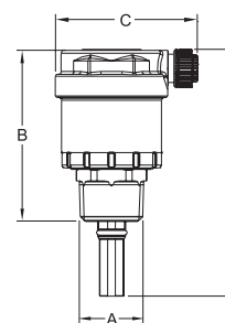
Modèle AVA-050 avec clapet anti-retour
