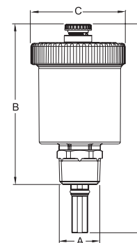
Modèle AVV-050 avec clapet anti-retour
