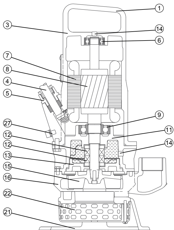
DRF 75-100/2/G40V DRF 150-200/2/G50V-G65V
