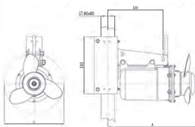
TBX 1.5 / 6E ET TBX 2.2 / 6E
