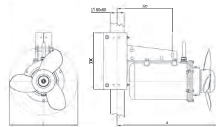
TBX 3 / 6E ET TBX 4 / 6E
