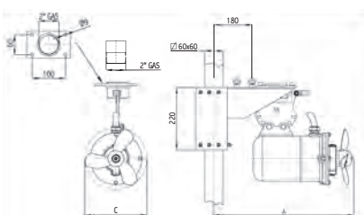
TBX 0.75 / 4E ET TBX 1.1 / 4E
