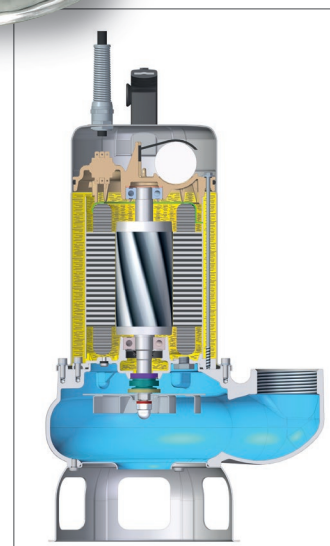
GIRANTE - IMPELLER
