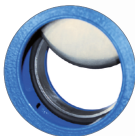
Siège interchangeable (NBR, EPDM, FKM, SILICONE, PTFE)
