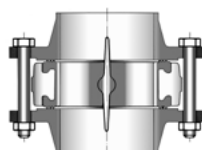
Serrage des boulons robinet ouvert
