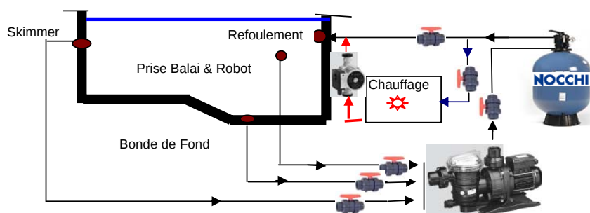
Shéma d'installation
