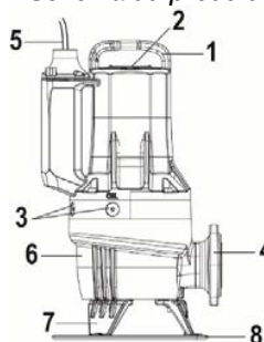
Fig. 2 Pompe FX RANGE
