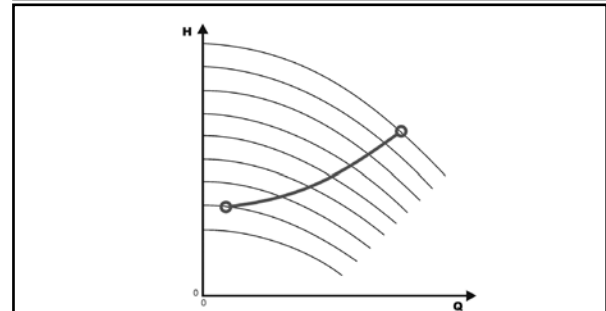
Contrôle pour correspondre à une courbe de système
