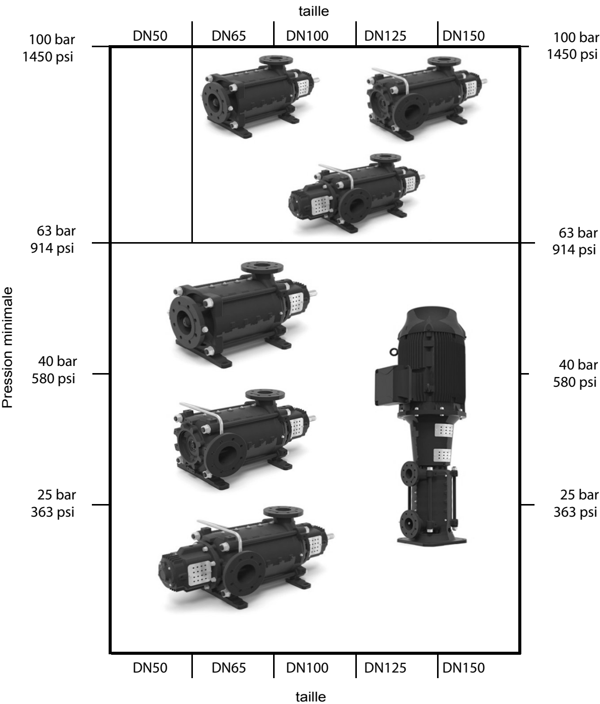
Plage de fonctionnement par taille et configuration
