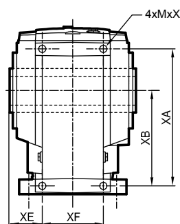
Ot arbre creux H
