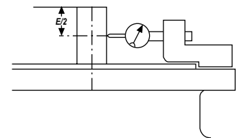
① Mesure de battement ou faux-rondu du bout d'arbre des moteurs à bride
