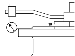
② Mesure de la concentricité du diamètre d'emboîtement
