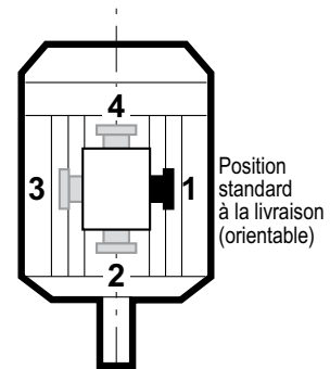
Position 2 peu recommandée (irréalisable sur moteur standard à bride à trous lisses FF)
