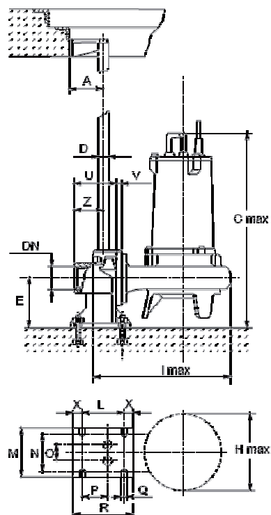
Dimensions caractéristiques
