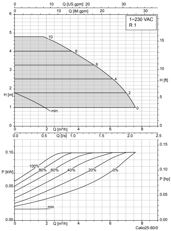
Calio 25-60, Δpc
