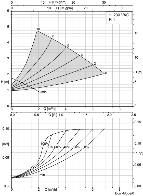
Calio 25-60, EcoMode
