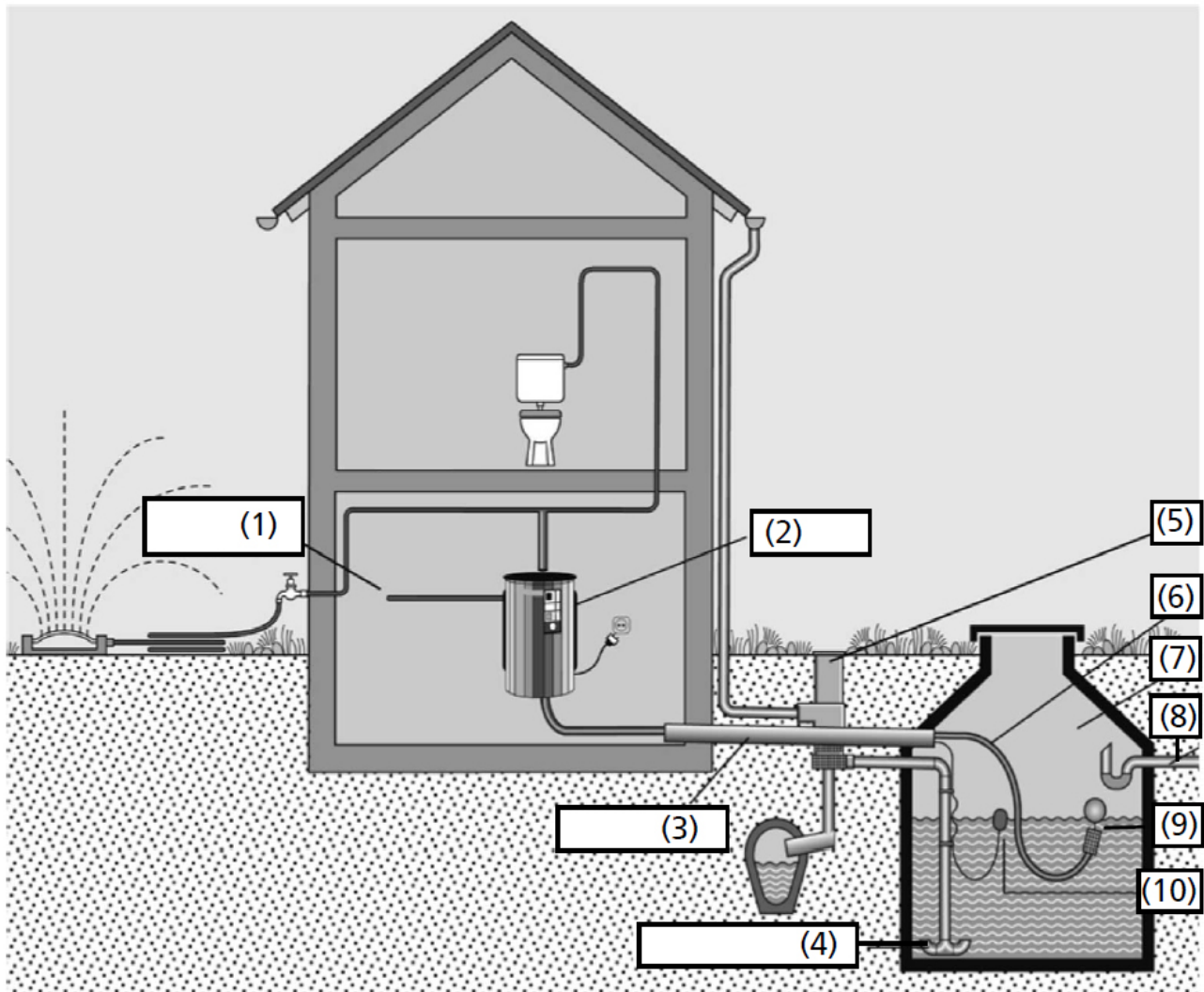
Schéma d'installation avec citerne enterrée à l'extérieur du bâtiment
