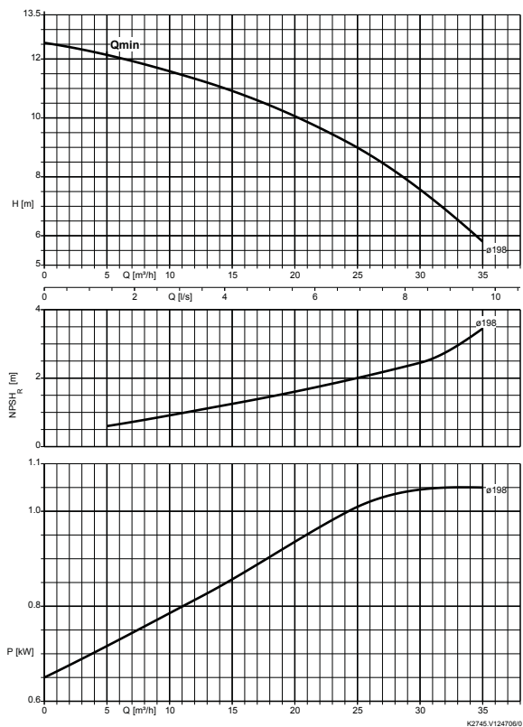
Etaprime 80-200, n = 1450 min -1
