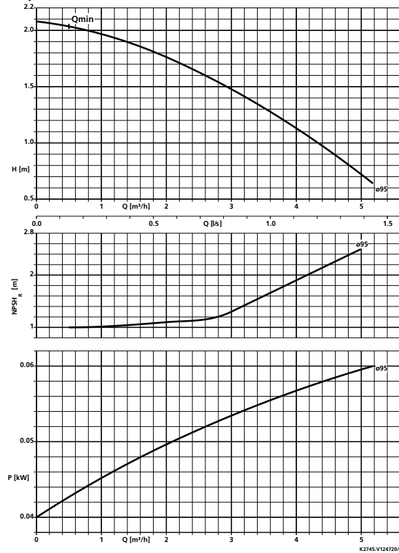
Etaprime 25-100, n = 1450 min -1
