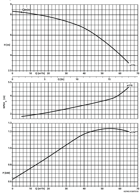
Etaprime 80-190, n = 1450 min -1
