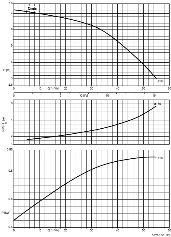
Etaprime 80-170, n = 1450 min -1
