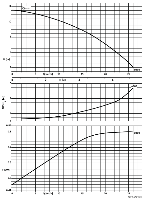
Etaprime 40-110, n = 2900 min -1
