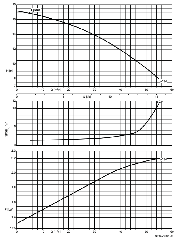
Etaprime 100-240.1, n = 1450 min -1
