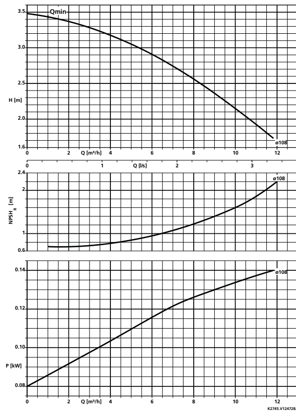
Etaprime 40-110, n = 1450 min -1
