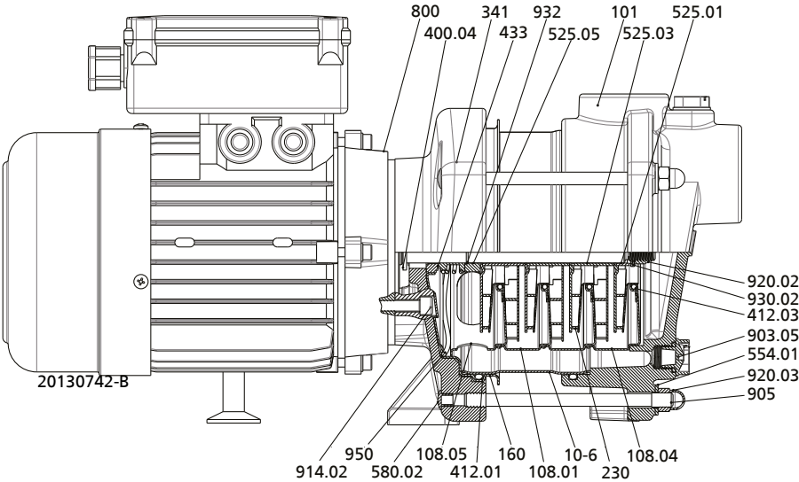
III. 3: Plan d'ensemble
