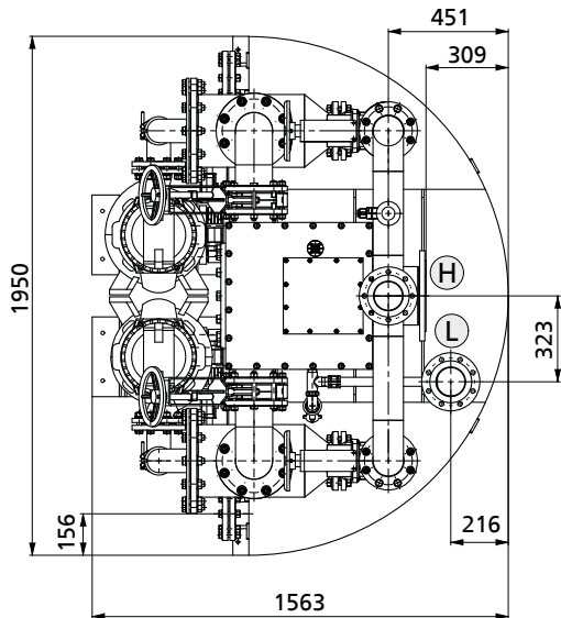
Dimensions, séparateur de matières solides (exemple) [mm]
