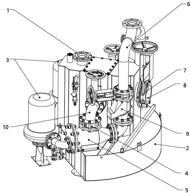
Schéma du séparateur de matières solides
