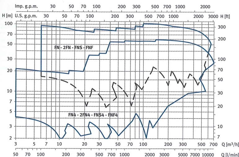
Plage de performance à 2900 rpm - Courbes répondant à la norme ISO 9906
