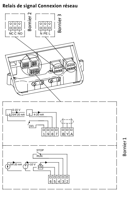
Fig. 28 Schéma de câblage en monophasé, TPE(D)
