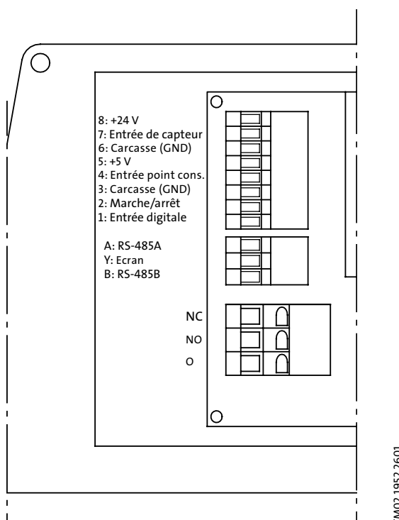
Fig. 30 Schéma de câblage en triphasé des TPE(D)
