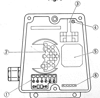
Boîte à bornes Vue de l'intérieur
