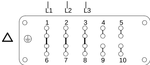
Fig. 37 Prises pour connexion triangle. Des éclisses de connexion sont situées dans la prise.
