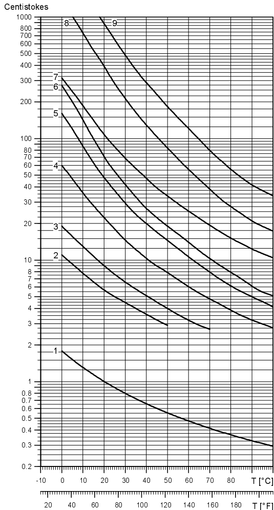
Fig. 48 Viscosité cinématique de plusieurs huiles par rapport à la température de l'huile
