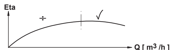
Fig. 40 Meilleure performance
