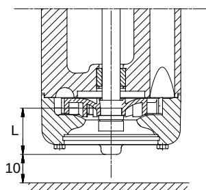
Fig. 29 Distance minimum entre la pompe et le réservoir
