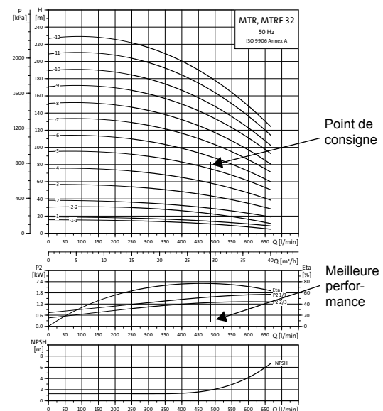
Fig. 39 Exemple d'un point de consigne d'une pompe MTR
