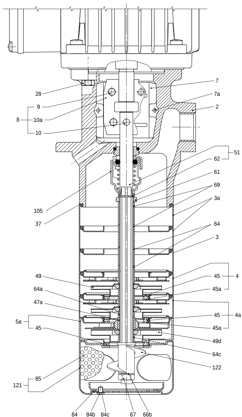
Fig. 12 SPK 1, SPK 2
