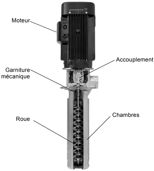
Fig. 3 Pompe MTR
