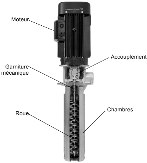
Fig. 4 Pompe SPK
