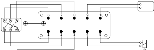
Fig. 35 Du moteur
