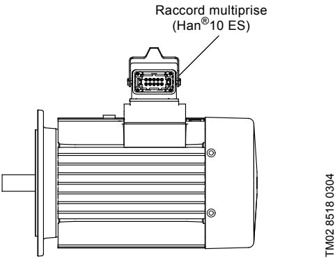
Fig. 33 Multiprise type Han® 10 ES
