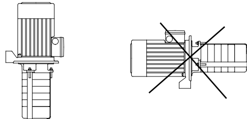
Fig. 26 Installation d'une pompe MTH
