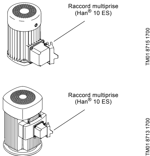
Fig. 32 Multiprise sur un moteur Grundfos MG
