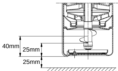
Fig. 25 SPK, SPKE
