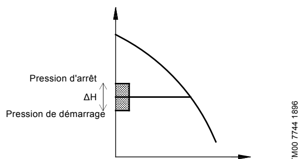
Fig. 10 Pressions de démarrage et d'arrêt
