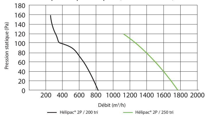
Hélipac® 3 triphasé - 2 pôles (mural et tubulaire)
