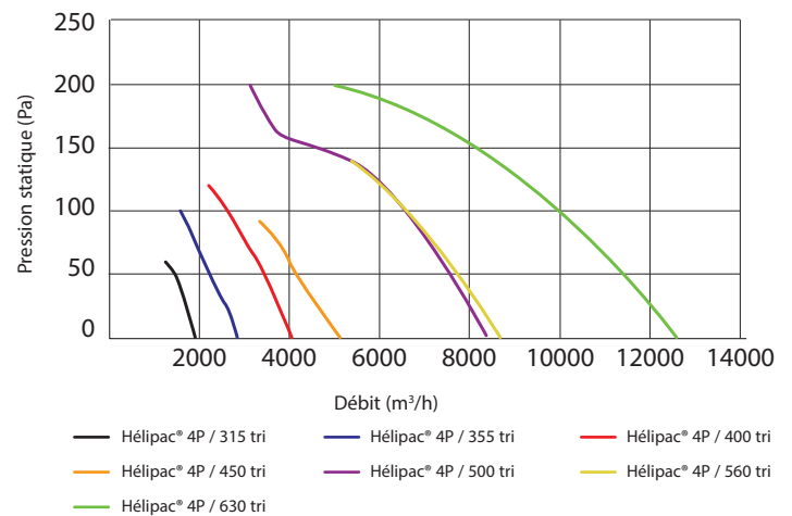
Hélipac® 3 triphasé - 4 pôles (mural et tubulaire)
