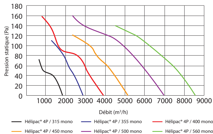
Hélipac® 3 monophasé - 4 pôles (mural et tubulaire)
