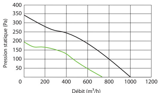
Canal Fast® isolé 200
