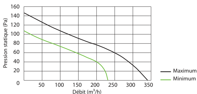
Canal Fast® isolé 150
