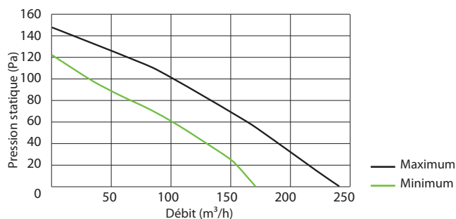
Canal Fast® isolé 125
