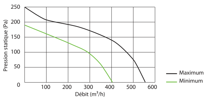
Canal Fast® isolé 200
