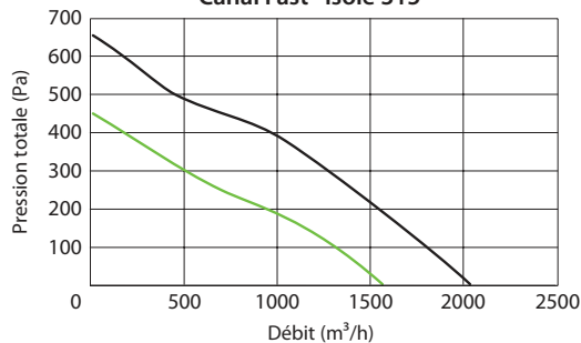
Canal Fast® isolé 315 S et 400
