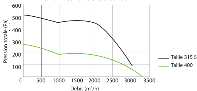
Canal Fast® isolé 315 S et 400
