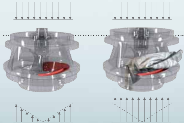
Fig. 1 : répartition des efforts en fonctionnement normal
