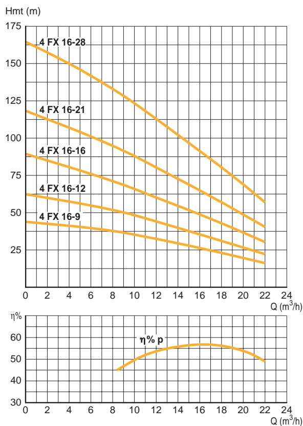
Courbes de Performances Série 4 FX 16
