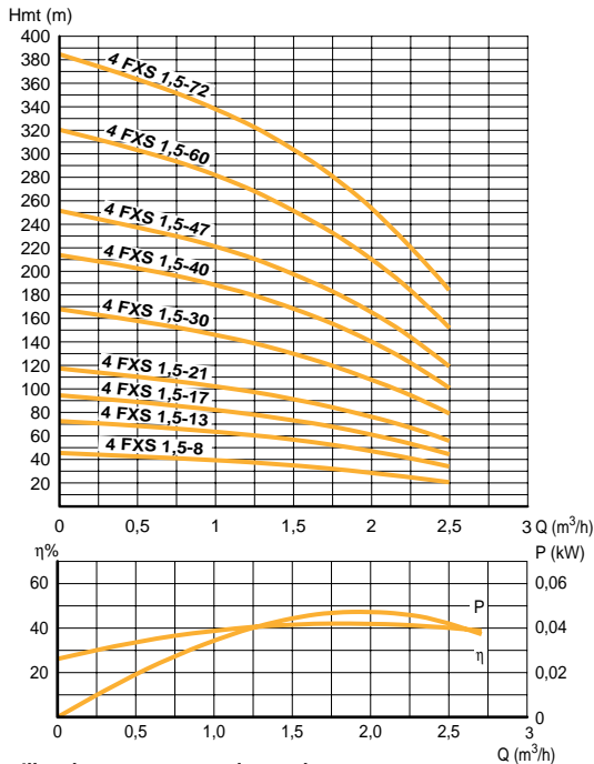
Courbes de performances Série 4 FXS 1,5
