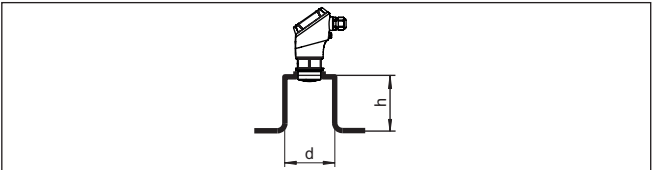
Fig. 11: Montage sur rehausse
