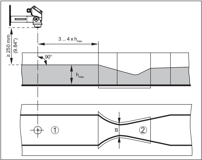
Fig. 18: Mesure du débit avec canal Venturi Khafagi : h_{max} = remplissage max. du canal ; B = resserrement max. du canal
