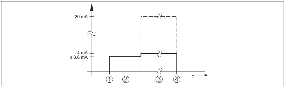
Fig. 34: Durée de démarrage et édition de valeur de mesure
