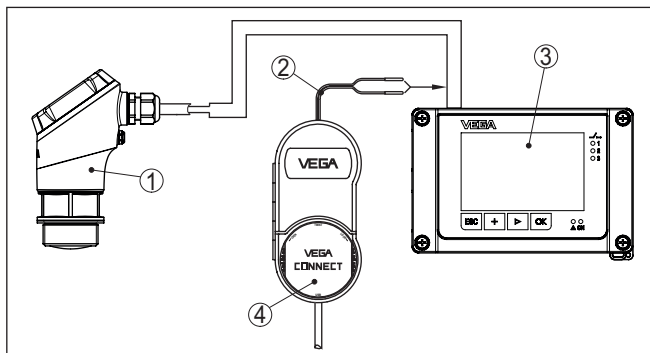
Fig. 30: Raccordement du PC à l'unité de commande VEGAMET
