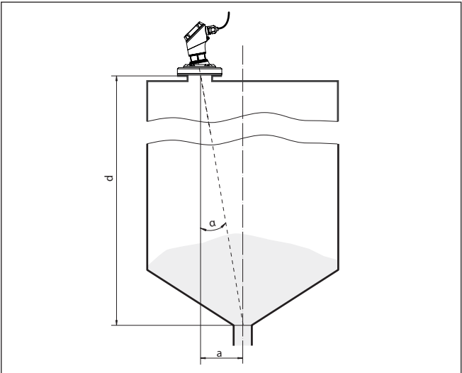
Fig. 15: Proposition pour un montage après orientation VEGAPULS 31
