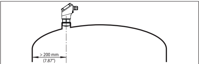
Fig. 7: Montage du capteur radar dans une cuve à toit bombé
