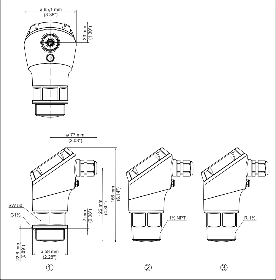
Fig. 36: Encombrement VEGAPULS 31
