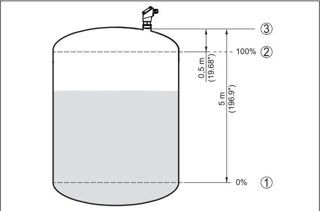
Fig. 24: Exemple de paramétrage réglage min./max.
