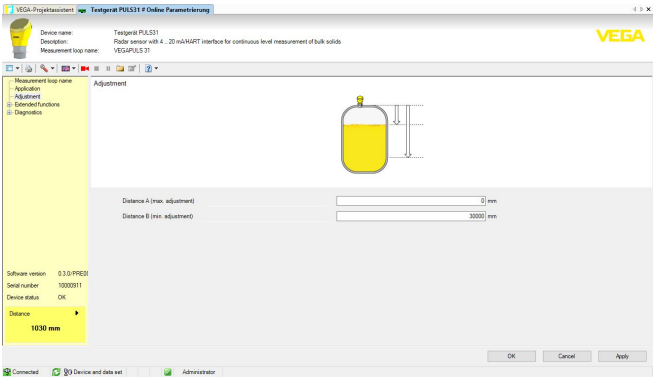
Fig. 28: Exemple de vue DTM - Mise en service réglage du capteur
