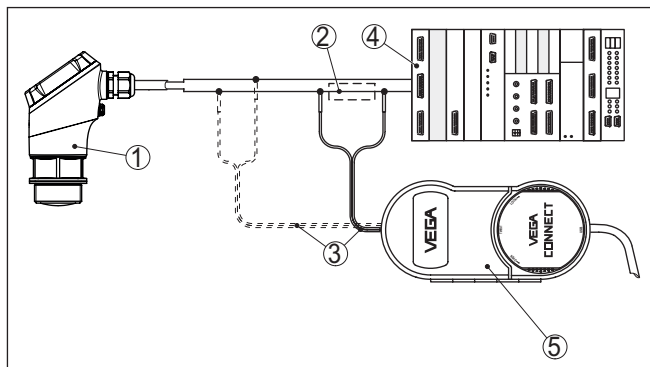
Fig. 29: Raccordement du PC à la ligne signal
