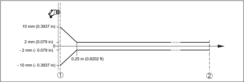
Fig. 35: Écart de mesure sous conditions de référence 10)
