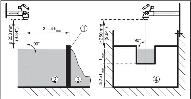
Fig. 17: Mesure du débit avec déversoir rectangulaire: h_{max} = remplissage max. du déversoir rectangulaire
