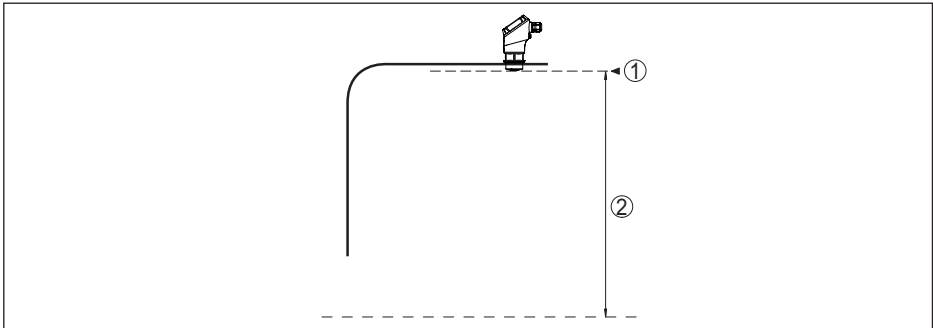
Fig. 33: Données relatives à la grandeur d'entrée
