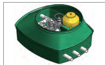
Ballon anti-bélier dans le regard pour protéger les systèmes de pompage et le réseau de refoulement
