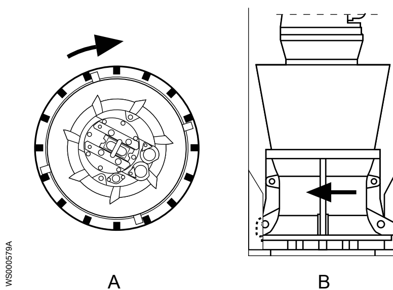
Рис. 35: Вид сверху (A) и вид сбоку (B)
