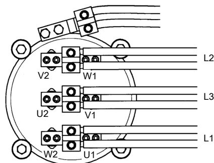
Рис. 23: 2 кабеля, приводы 805/815, 835/845, 865/875, 885/895; 905/915, 935/945, 965/975; 705/715, 735/745, 765/775
