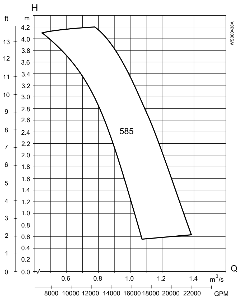
Рис. 65: P7076, 60 Гц, низкое напряжение
