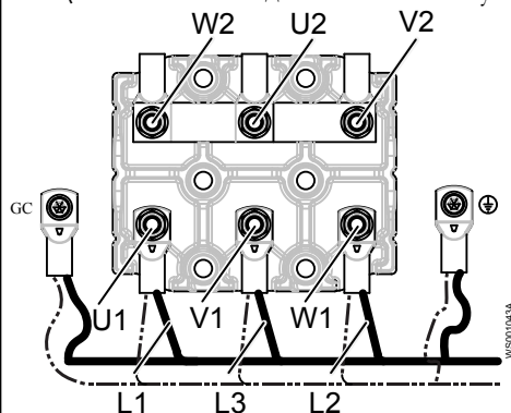
Рис. 26: Приводы 605/615, 665/675; 705/715, 735/745, 765/775
