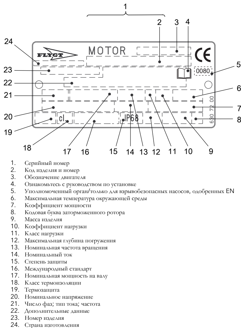
Рис. 5: Табличка для приводного блока начиная с 990101
