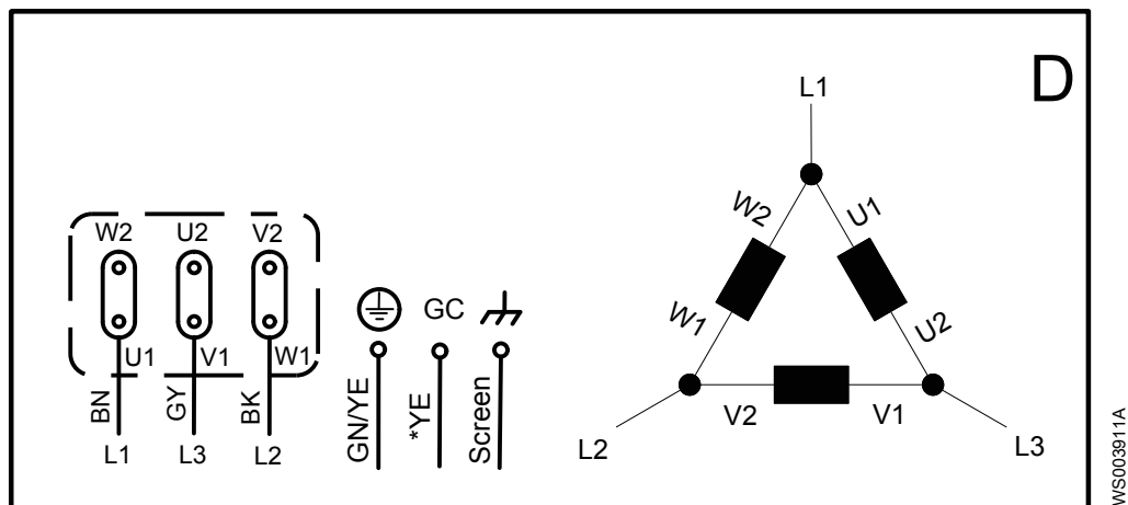
Рис. 24: Схема
