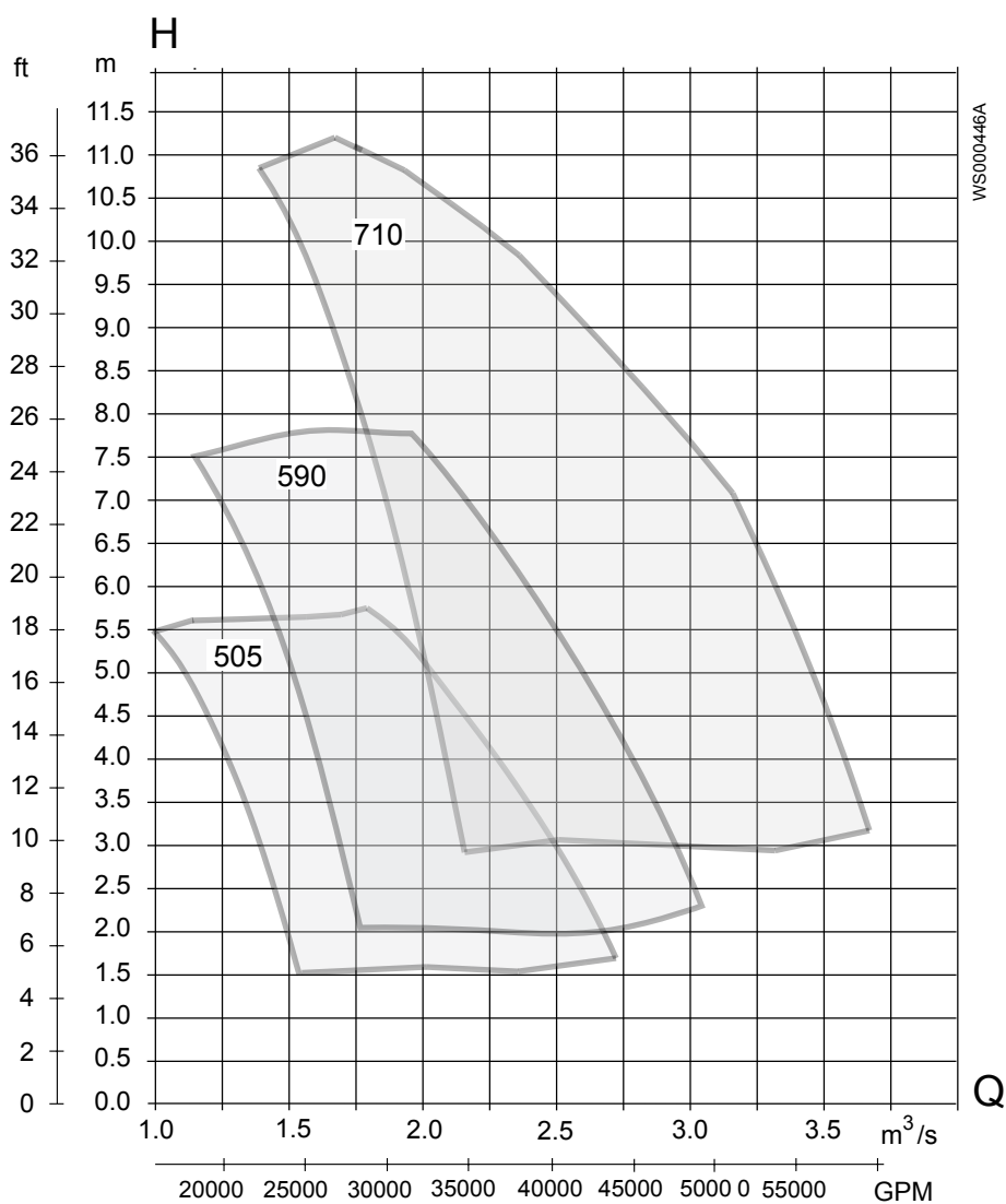
Рис. 17: P7101, 60 Hz, среднее напряжение
