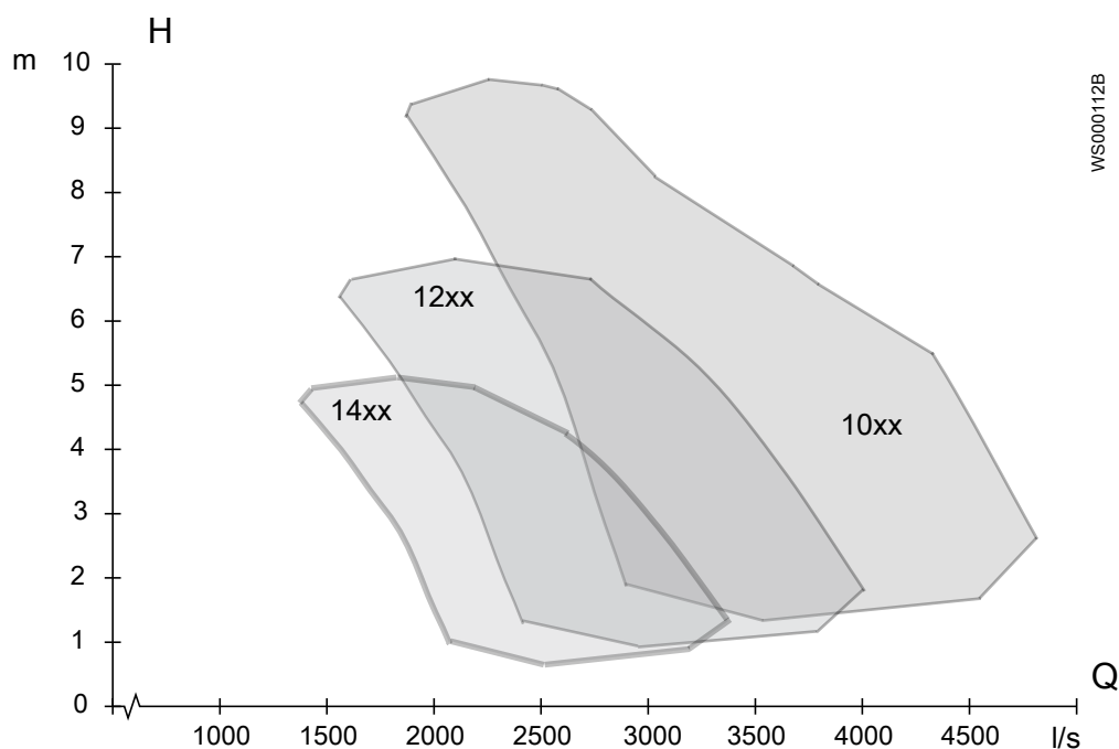
Рис. 6: P7105, 50 Гц, низкое напряжение
