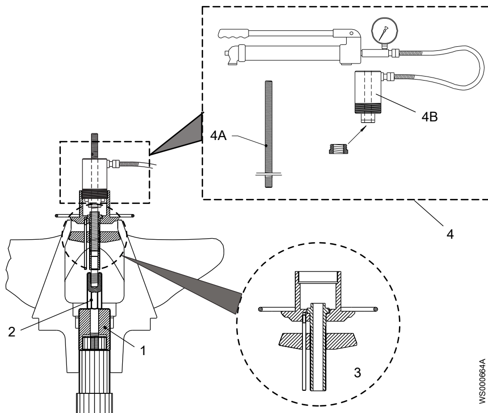
Рис. 37: Инструменты и детали, необходимые для снятия пропеллера
