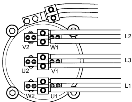
Рис. 17: Соединения, 2 кабеля, приводы 805/815, 835/845, 865/875, 885/895
