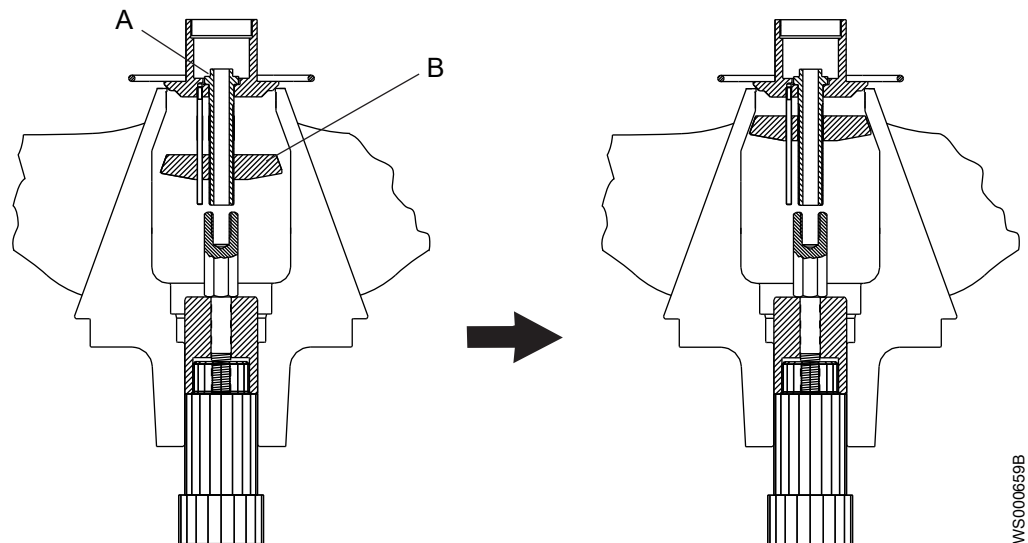
Рис. 39: Монтаж съемника
