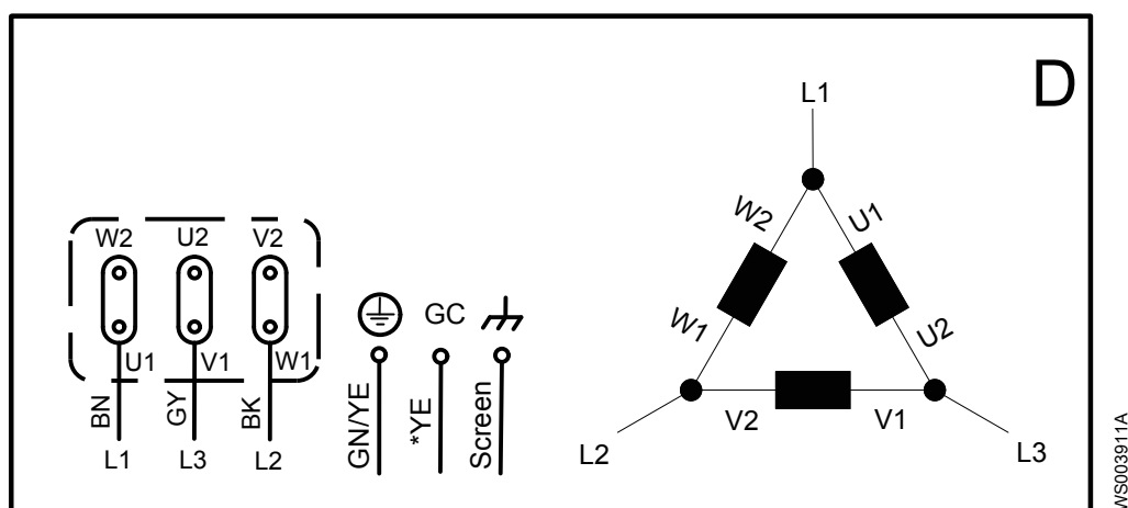
Рис. 16: Схема
