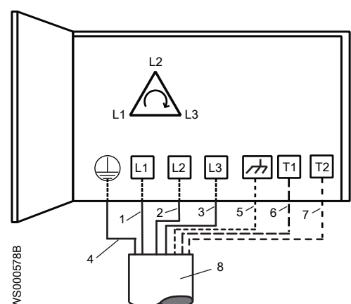
Рис. 8: Правильное чередование фаз
