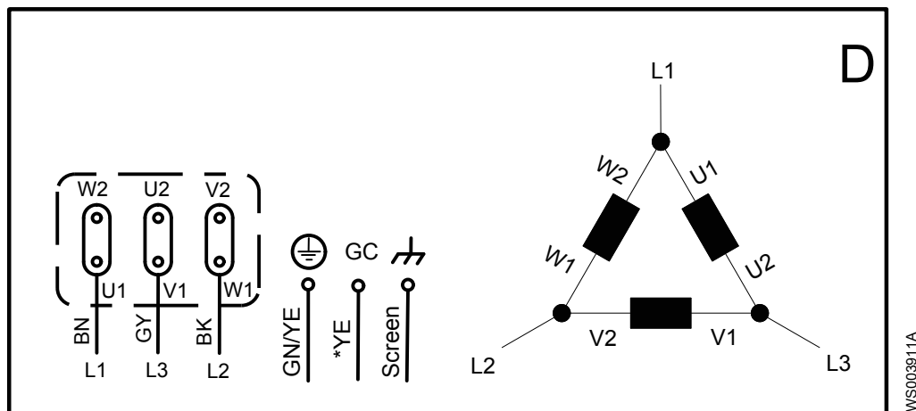
Рис. 18: Схема
