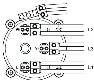
Рис. 15: Соединения, приводы 805/815, 835/845, 865/875, 885/895
