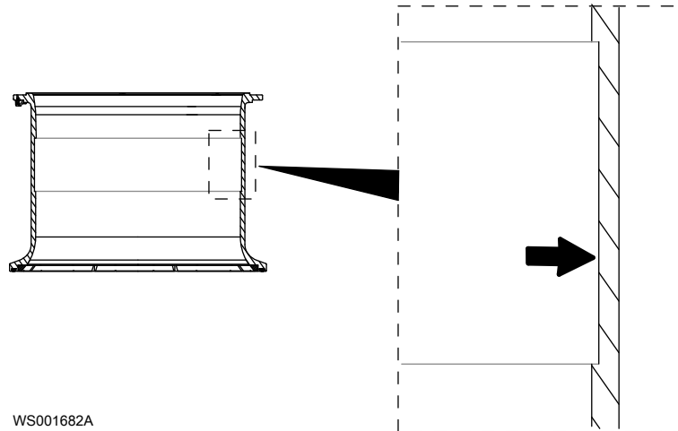
Рис. 36: Канавка для компенсационного кольца
