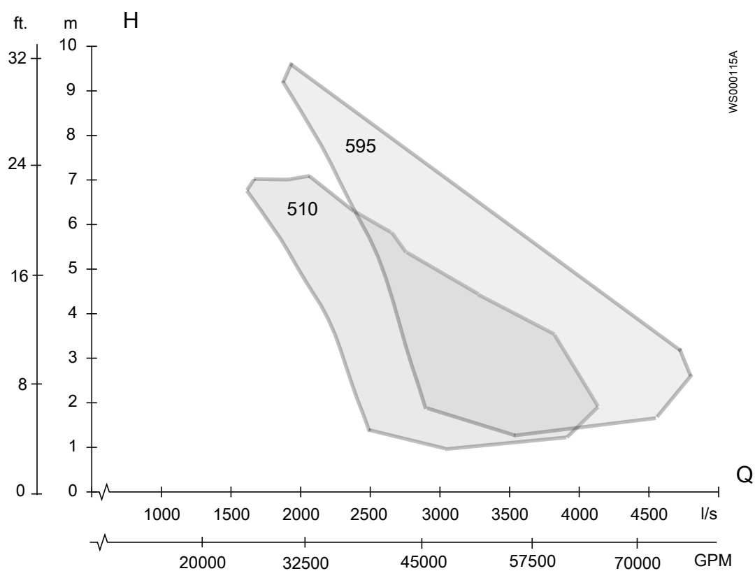
Рис. 47: P7105, 60 Гц, среднее напряжение
