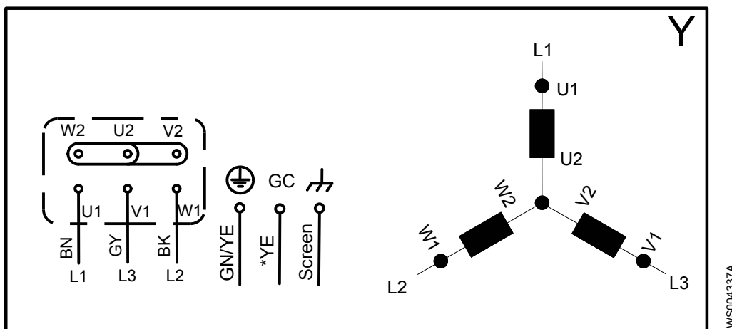
Рис. 20: Схема
