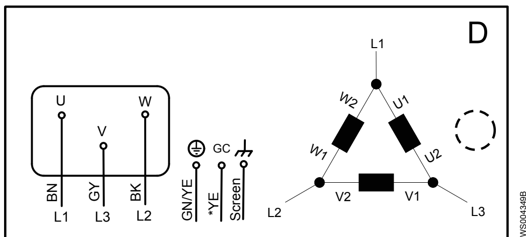
Рис. 14: Схема
