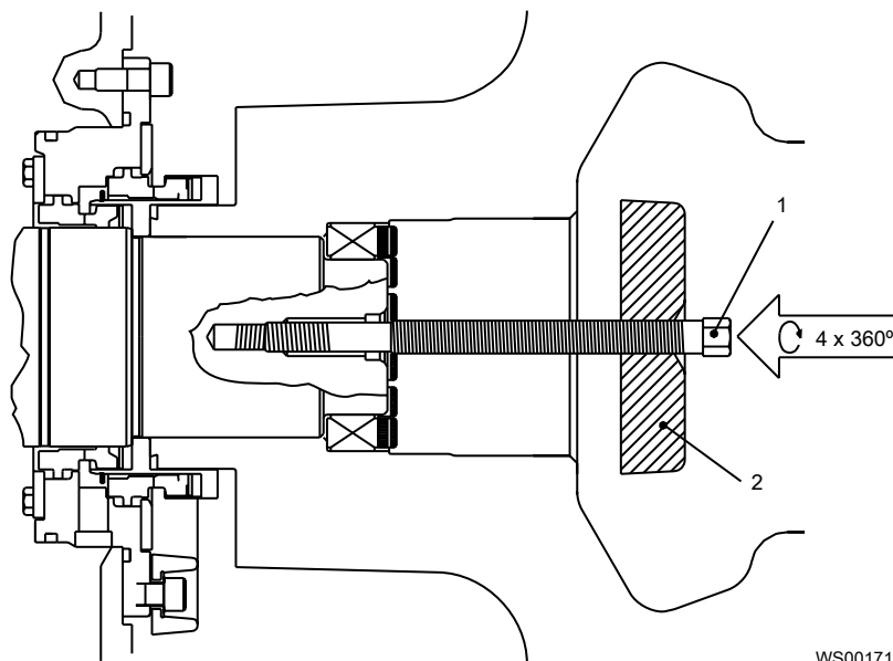
Рис. 42: Механизм блокировки в сборе
