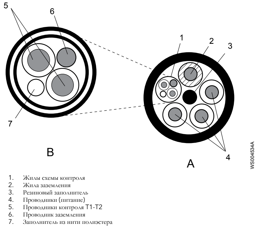
Рис. 29: Пример кабеля SUBCAB с жилами питания и управления
