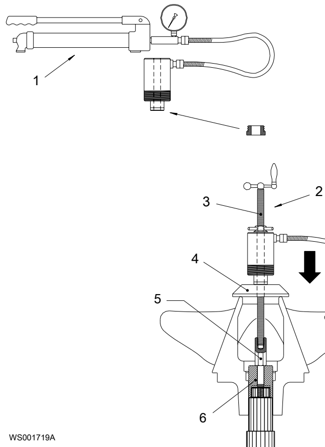
Рис. 41: Установка рабочего колеса на место, P7105
