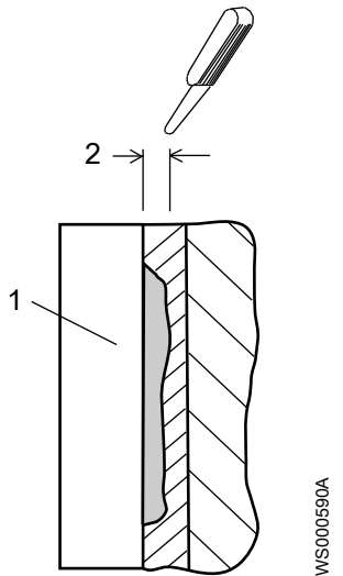
Рис. 34: Измерение износа компенсационного кольца
