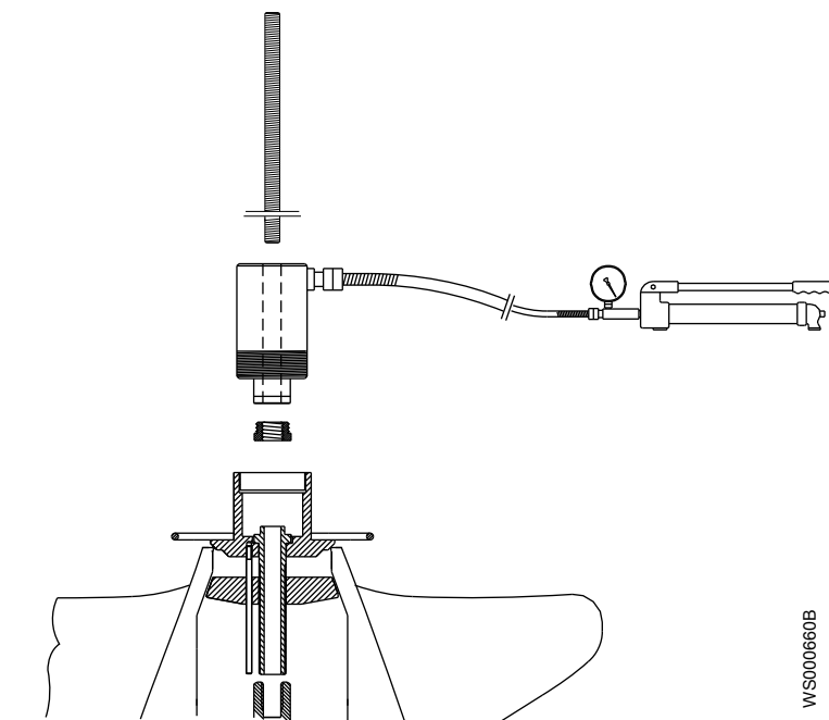
Рис. 40: Установка гидравлического инструмента и резьбового стержня.
