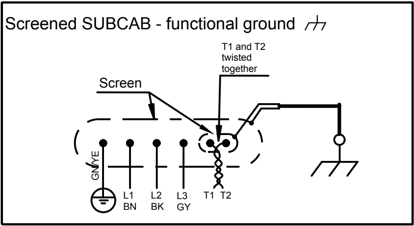
Рис. 27: С функциональным заземлением
