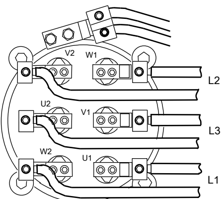
Рис. 23: Соединения, приводы 805/815, 835/845, 865/875, 885/895
