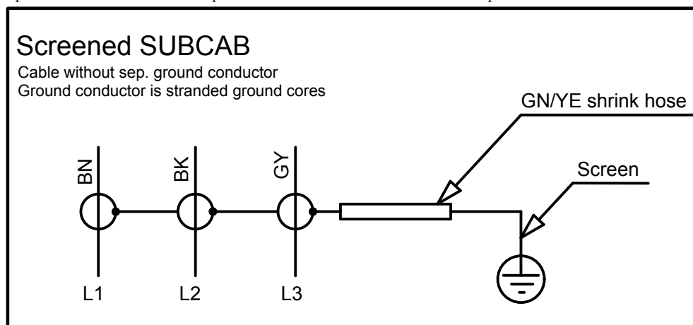
Рис. 26: Без отдельного проводника заземления
