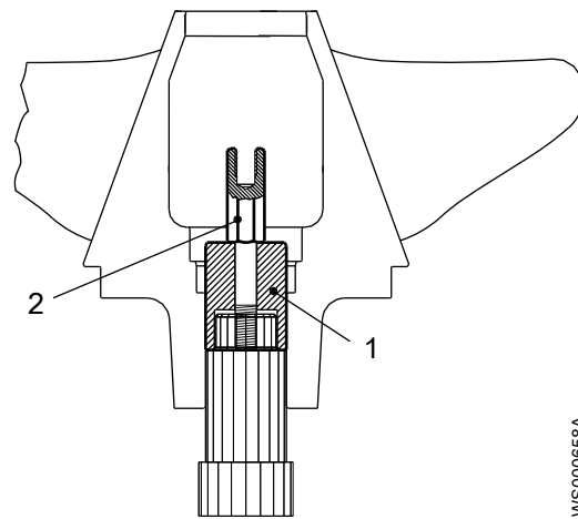
Рис. 38: Монтаж втулки и распорного винта
