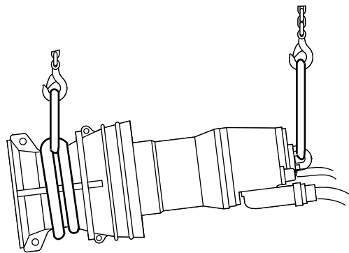
Рис. 32: Поднимание агрегата для ремонтных работ (показан типичный агрегат)
