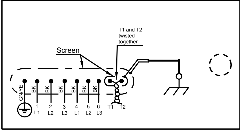
Рис. 28: С функциональным заземлением
