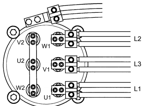
Рис. 21: Соединения, приводы 805/815, 835/845, 865/875, 885/895
