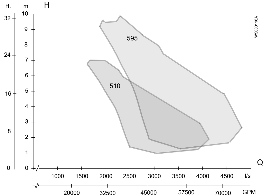
Рис. 46: P7105, 60 Гц, низкое напряжение
