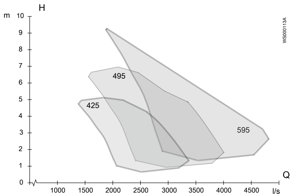
Рис. 45: P7105, 50 Гц, среднее напряжение
