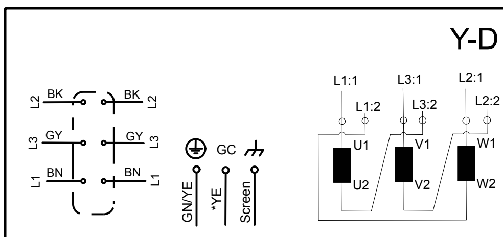
Рис. 22: Схема
