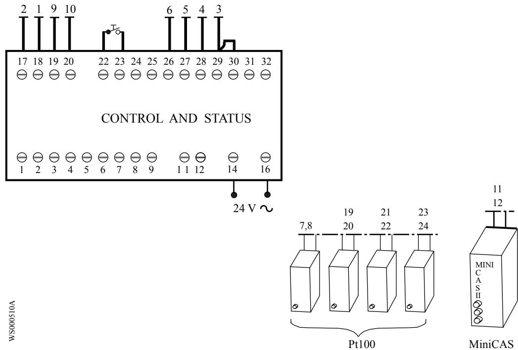
Рис. 13: Подключения к основному блоку CAS.
