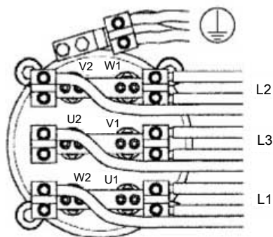
Рис. 19: Соединения, 3 кабеля, приводы 805/815, 835/845, 865/875, 885/895
