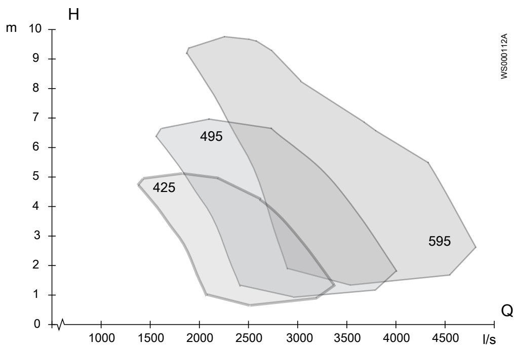
Рис. 44: P7105, 50 Гц, низкое напряжение
