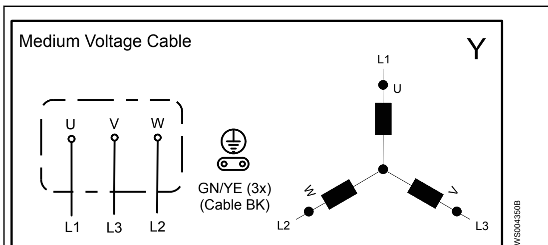
Рис. 24: Схема
