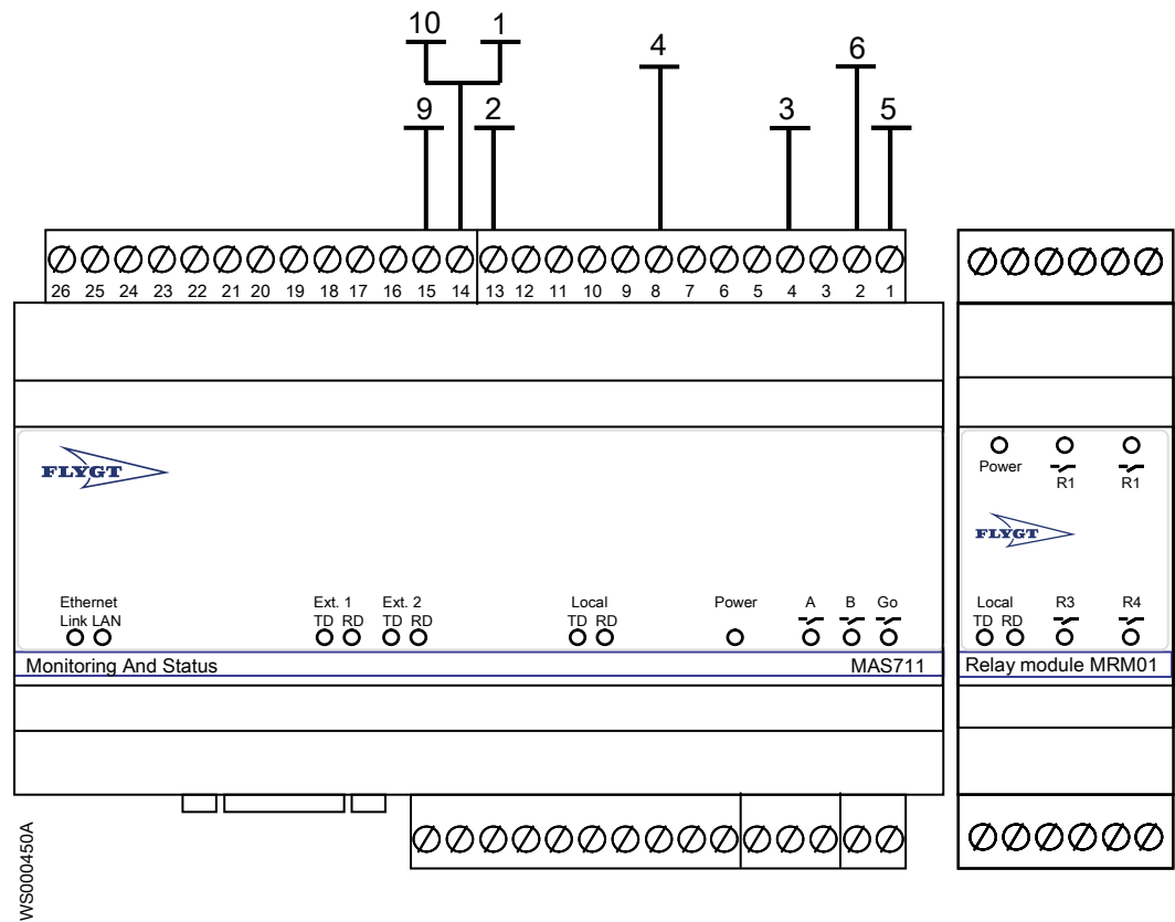
Рис. 12: Подключения к базовым блокам MAS 711 + MRM-01
