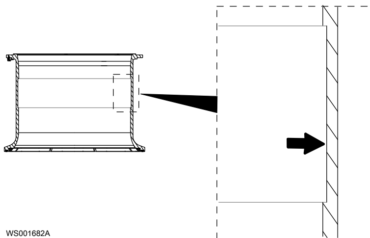
Рис. 41: Канавка для компенсационного кольца
