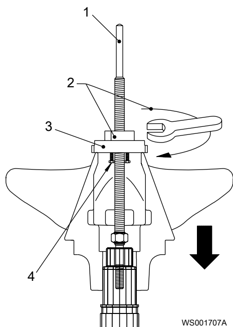
Рис. 43: P7065
