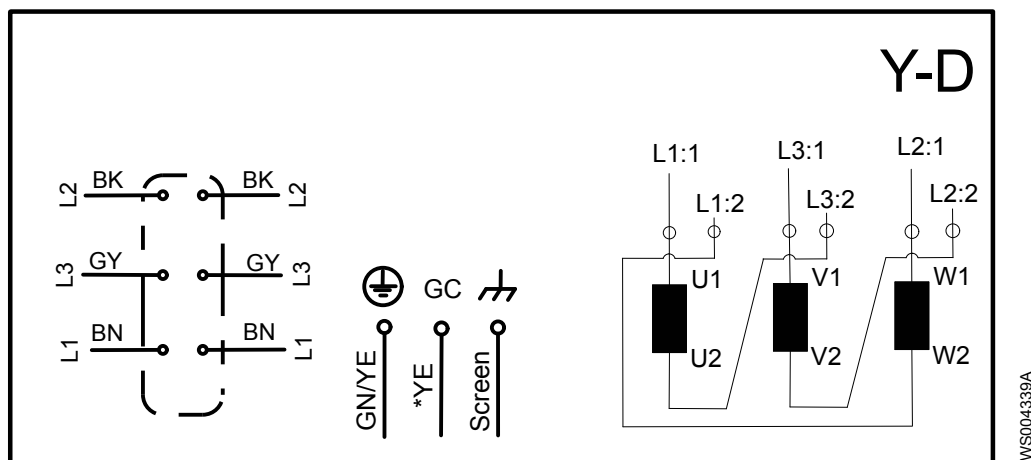
Рис. 28: Схема
