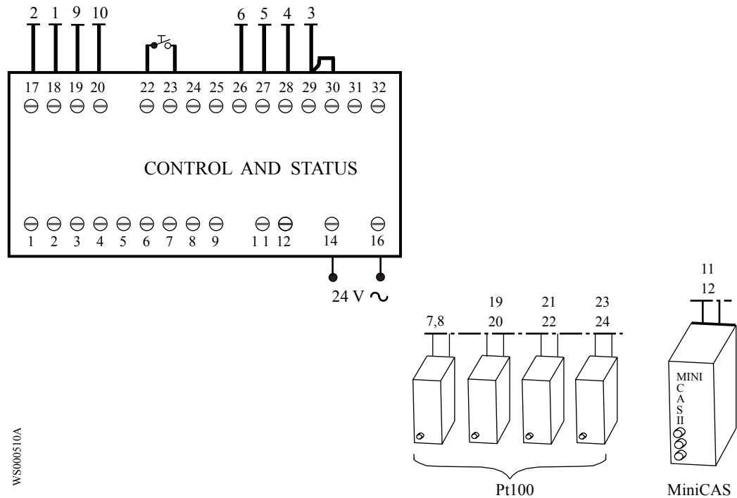
Рис. 14: Подключения к основному блоку CAS.
