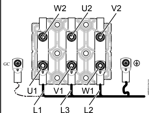
Рис. 19: Соединения, приводы 705/715, 735/745, 765/775
