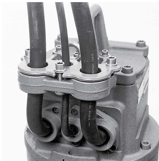
Рис. 8: Держатель кабеля
