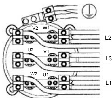
Рис. 24: Соединения, 3 кабеля, приводы 7X5 с большой соединительной коробкой
