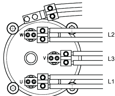
Рис. 17: Соединения, приводы 7X5 с большой соединительной коробкой
