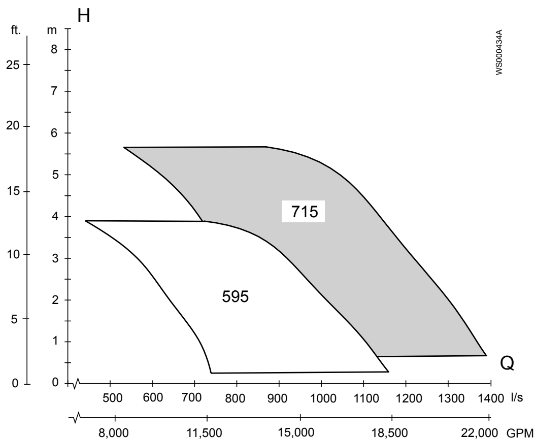
Рис. 46: P7065, 60 Гц, низкое напряжение, кривые 595 и 715
