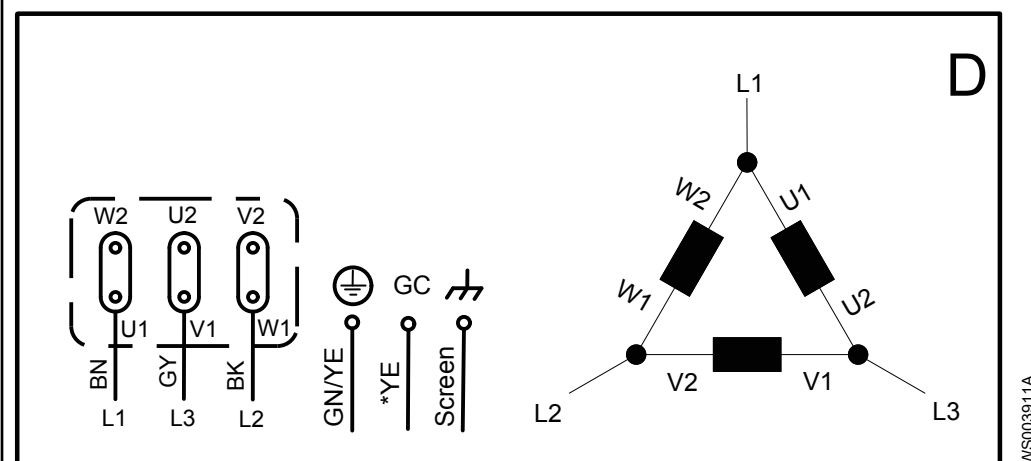
Рис. 18: Схема
