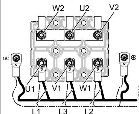
Рис. 26: Соединения, приводы 705/715, 735/745, 765/775
