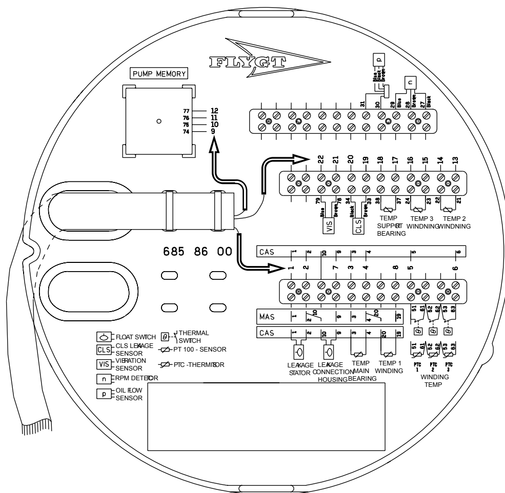
Рис. 10: Подключения к насосу. Стрелки указывают номера проводов кабеля SUBCAB.
