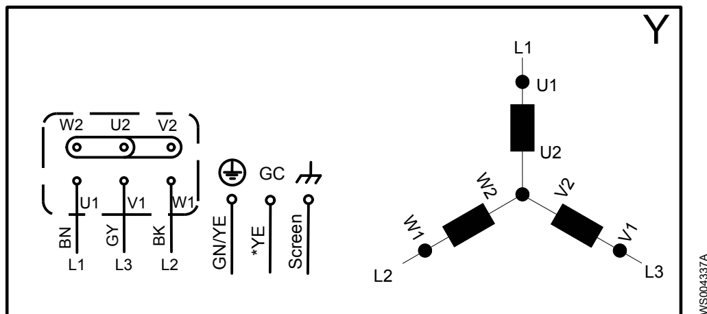
Рис. 25: Схема
