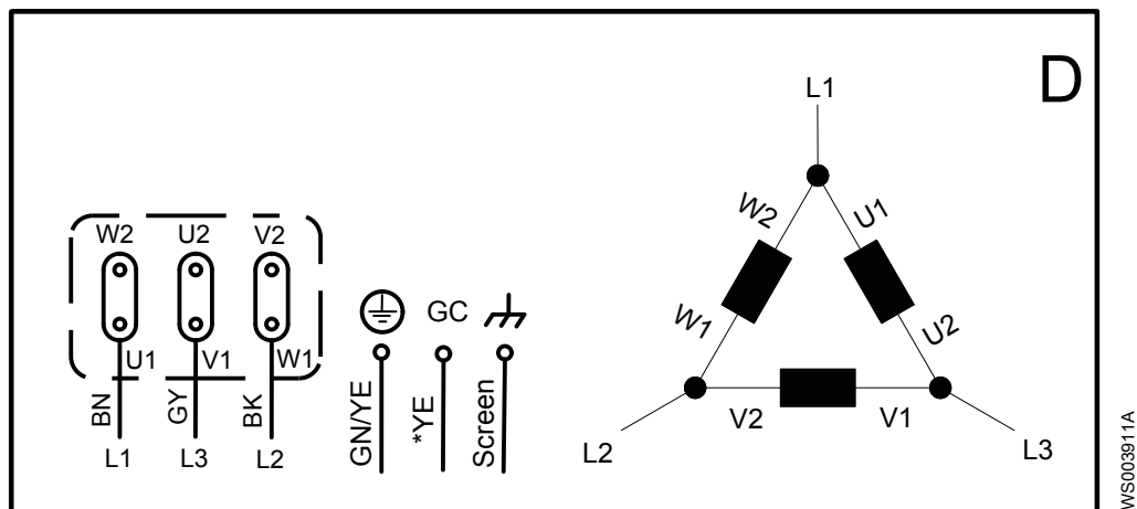
Рис. 23: Схема
