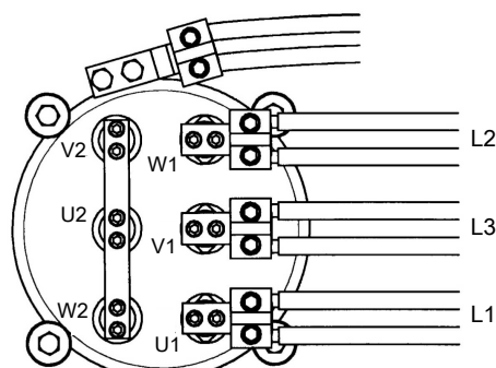
Рис. 27: Соединения, приводы 7X5 с большой соединительной коробкой
