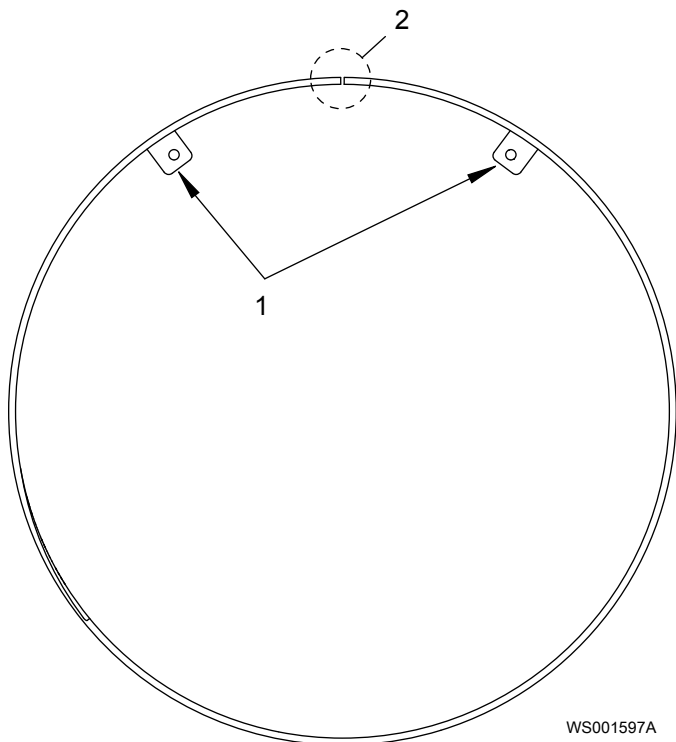
Рис. 40: Пластина толщиной 6 мм с крепежными выступами
