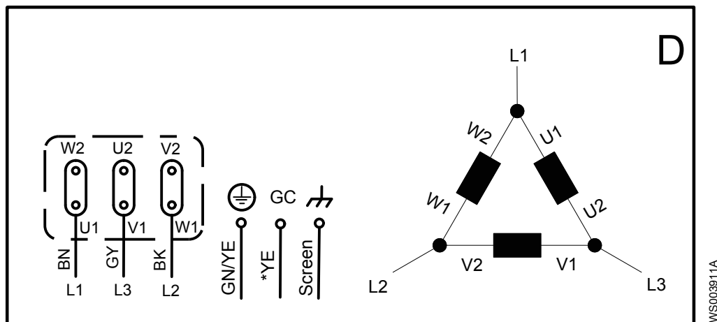
Рис. 20: Схема
