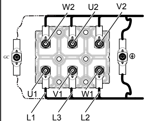
Рис. 29: Соединения, приводы 705/715, 735/745, 765/775
