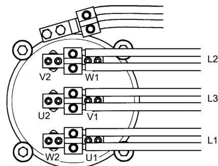
Рис. 22: Соединения, 2 кабеля, приводы 7X5 с большой соединительной коробкой
