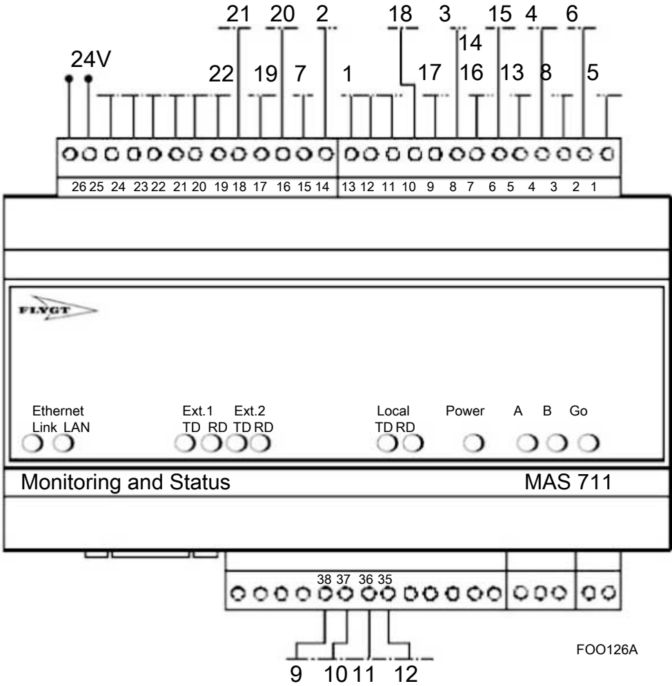
Рис. 11: Подключения к основному блоку MAS 711.
