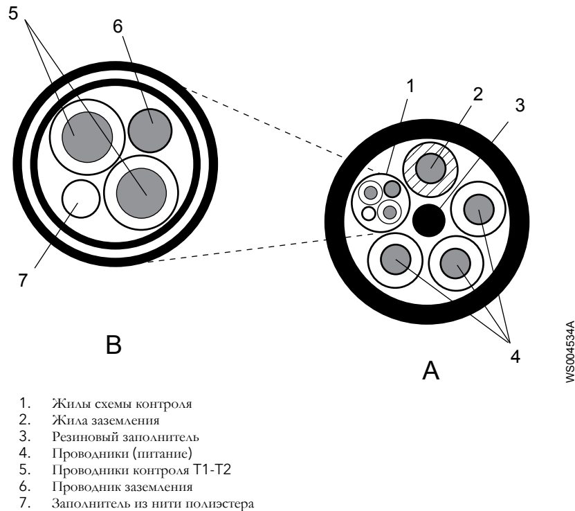
Рис. 34: Пример кабеля SUBCAB с жилами питания и управления
