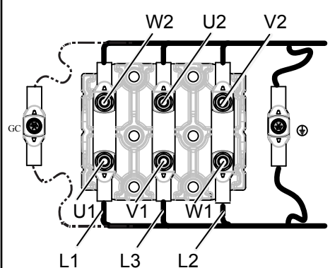
Рис. 21: Соединения, 2 кабеля, приводы 705/715, 735/745, 765/775
