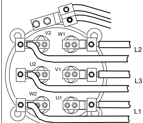
Рис. 30: Соединения, приводы 7X5 с большой соединительной коробкой
