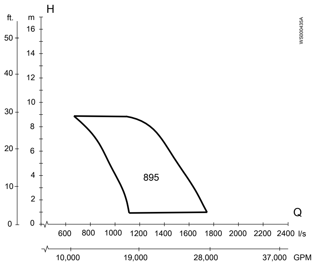
Рис. 47: P7065, 60 Гц, низкое напряжение, кривая 895
