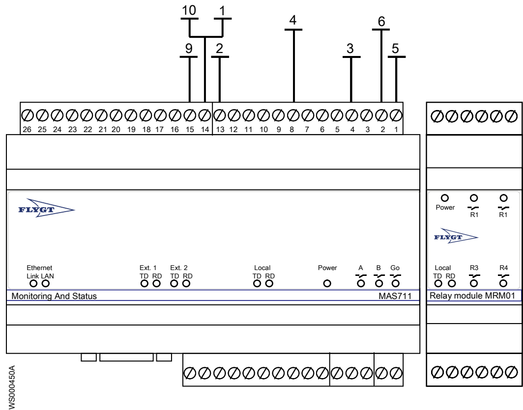
Рис. 13: Подключения к базовым блокам MAS 711 + MRM-01
