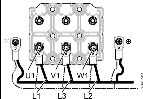
Рис. 16: Соединения, приводы 705/715, 735/745, 765/775
