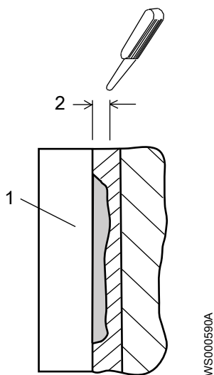
Рис. 39: Измерение износа компенсационного кольца
