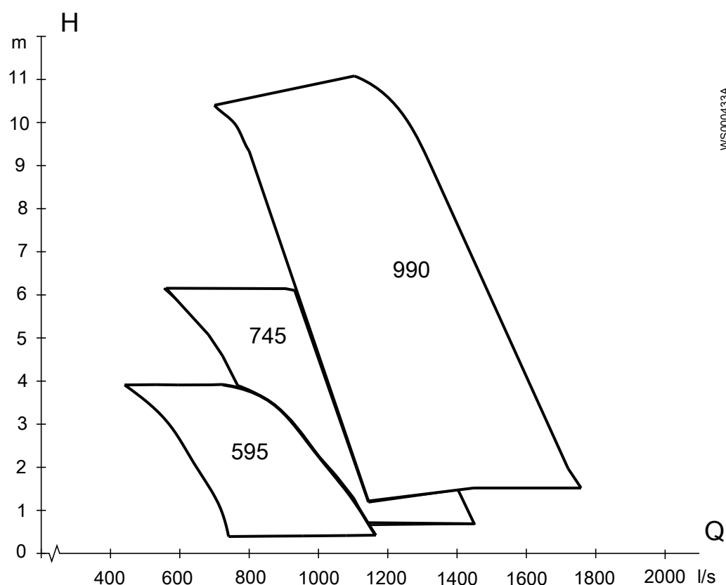
Рис. 45: P7065, 50 Гц, низкое напряжение
