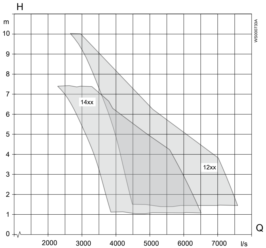
Рис. 11: P7125, 50 Гц, среднее напряжение
