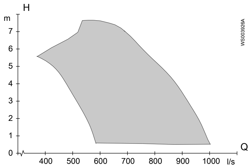
Рис. 4: P7040, 50 Гц
