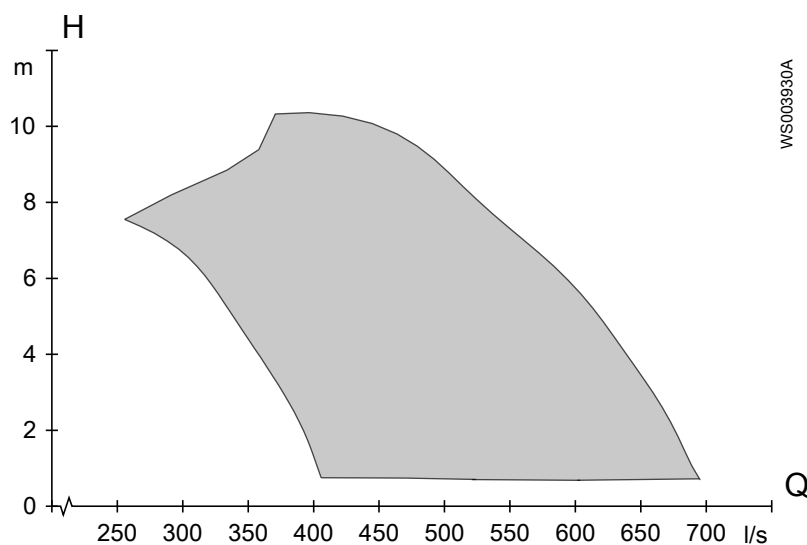
Рис. 3: P7035, 50 Гц
