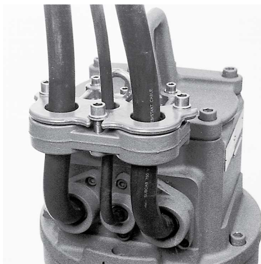
Рис. 10: Держатель кабеля
