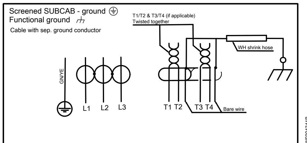
Рис. 26: С действующим заземлением
