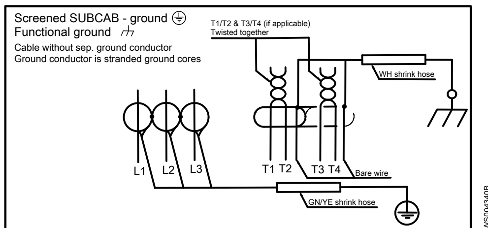
Рис. 25: Без отдельной жилы заземления.
