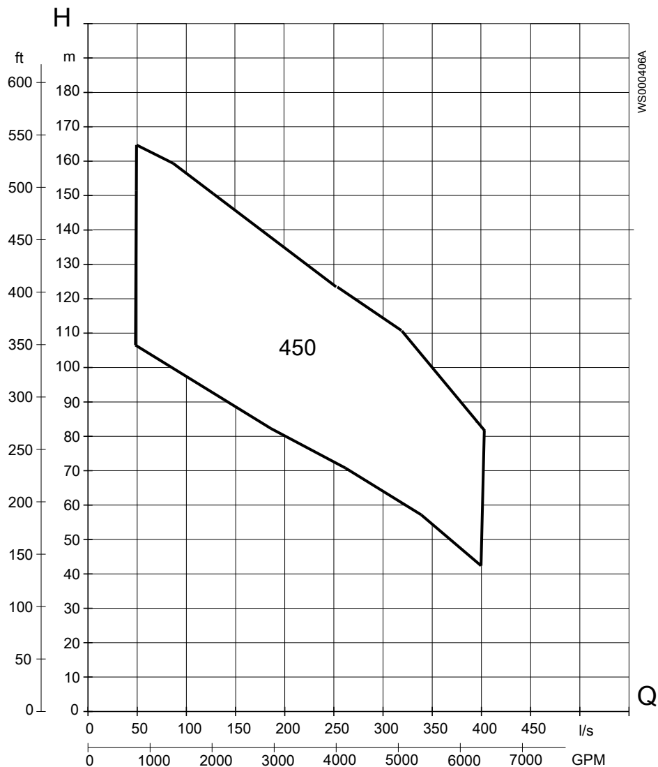
Рис. 21: C3240, 60 Hz, низкое напряжение
