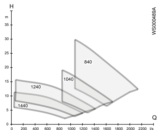
Рис. 16: С3602, 50 Нз, низкое напряжение
